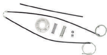
CÓD. 0106 - REPARO AUDI A3 4 PORTAS DIANTEIRAS - TODOS
