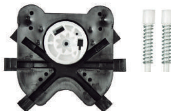
CÓD. 5148 - ADAPTADOR DA MÁQ. MANUAL P/ ELÉTRICA (C/ ROLD. MAREA, MOLAS E PONTEIRAS)
