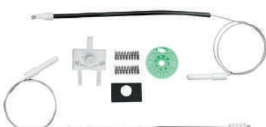
CÓD. 0139 - REPARO PALIO FIRE 4P, WEEKEND E SIENA DIANTEIRO ESQUERDO (ANO 1996 À 2017)
