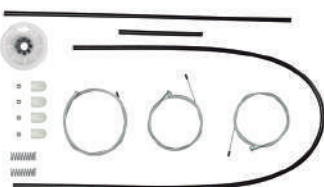
CÓD. 096 - REPARO PEUGEOT 207 PASSION 4 PORTAS DIANTEIRAS - TODOS
