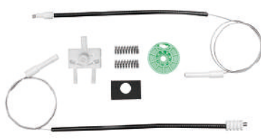
CÓD. 0138 - REPARO PALIO FIRE 4P, WEEKEND E SIENA DIANTEIRO DIREITO (ANO 1996 À 2017)
