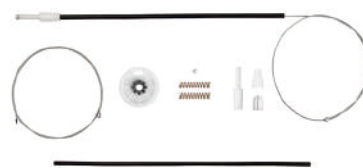
CÓD. 075 - REPARO RENAULT CLIO PORTAS DIANTEIRAS
